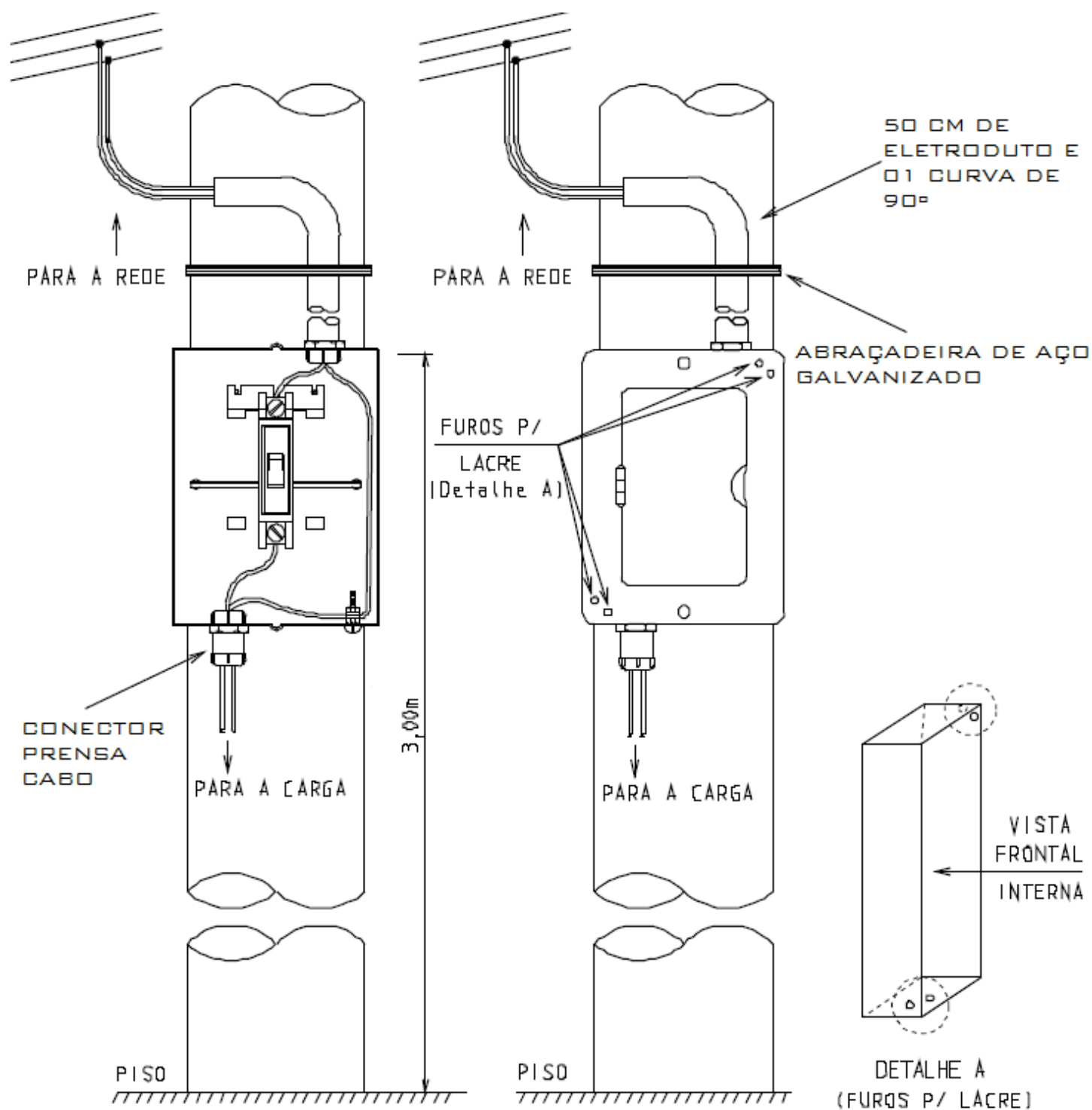
FIGURA 1 VISTA INTERNA DO QDG
