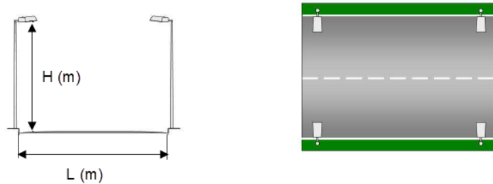
Figura 4: Posteamto bilateral frente a frente
