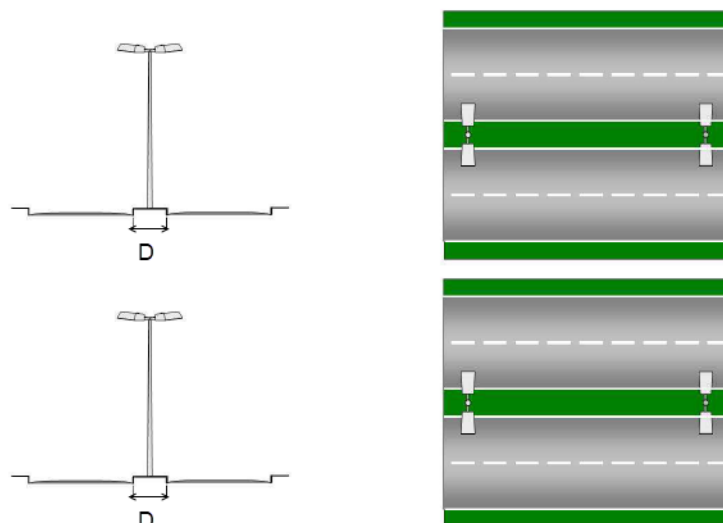
Figura 5: Posteamto no canteiro central
