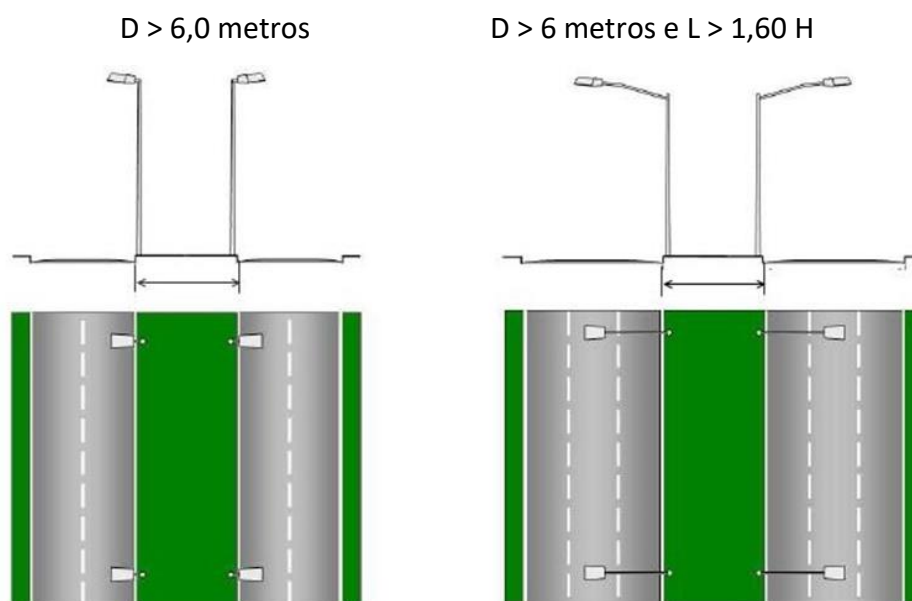
Figura 7: Posteamento central nos canteiros maiores que 6 metros
